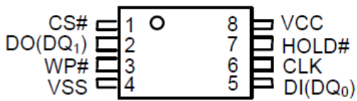
TDFN (2*3mm)
