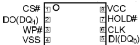
TDFN (2*3mm)
